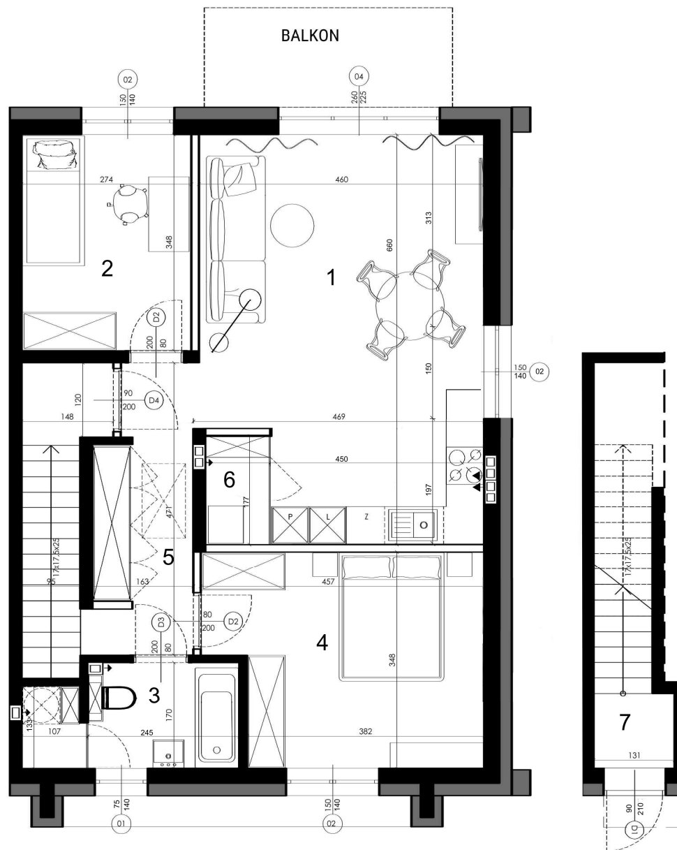
PIĘTRO
